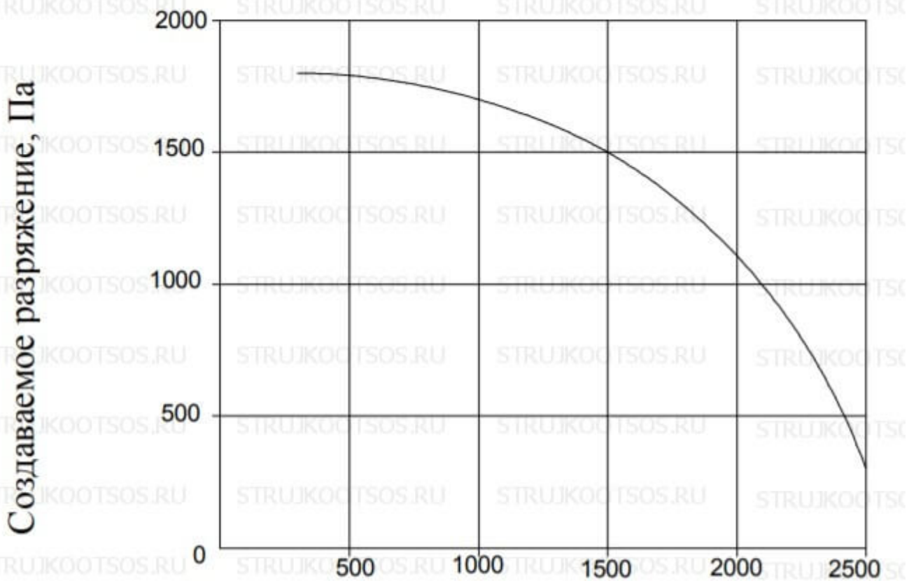
Производительность установки.
